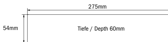
Lochausschnitt KME Einbaurahmen Hole cut-out KME recessed frame
