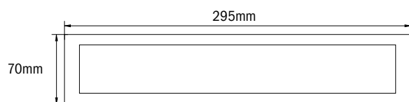
KME Einbaurahmen KME Recessed frame
