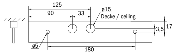
Maße KME Einbaurahmen Dimensions KME recessed frame
