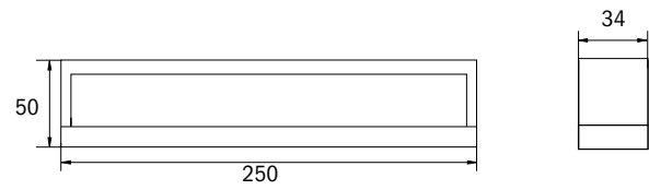
Lochausschnitt KME Einbaurahmen Hole cut-out KME recessed frame
