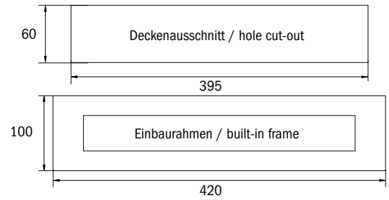
Lochausschnitt KE Einbau Hole cut-out KE recessed
