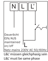
geschaltetes Dauerlicht
